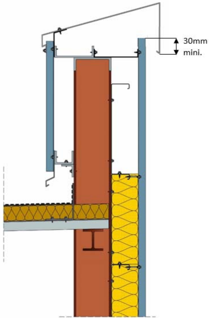
Figure 20 - Détail du haut de Bardage vertical
