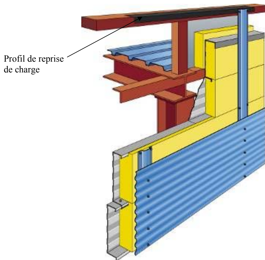
Figure 15 - Profil de reprise de charge filant fixé en haut de bardage
