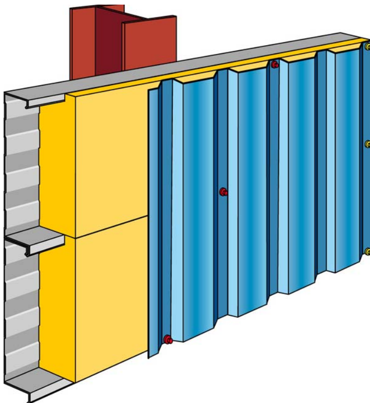
Figure 4 - Fixation SK-RB (Etanco) pour la fixation de l'Isobardage 32 en seconde couche
