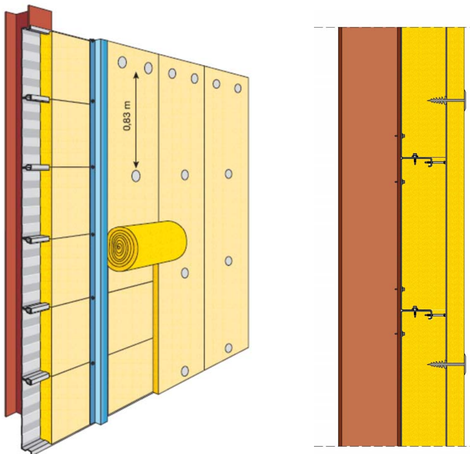
Figure 17 - Mise en œuvre d'une isolation en 2 couches
