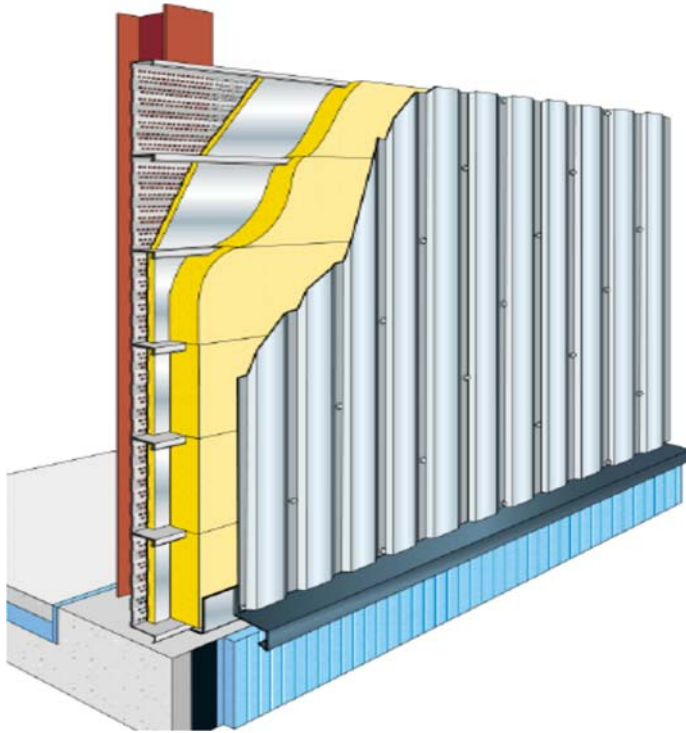
Figure 8 - Mise en œuvre de l'isolant Cladacoustic (Bardage vertical)
