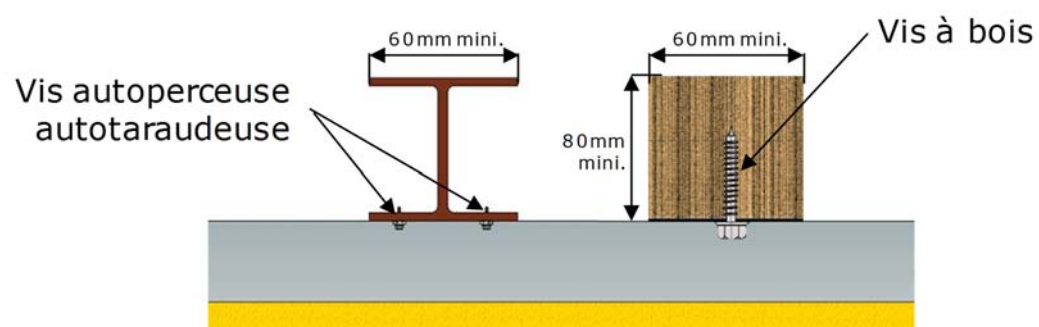
Figure 28 – Fixation des plateaux sur les différents supports
