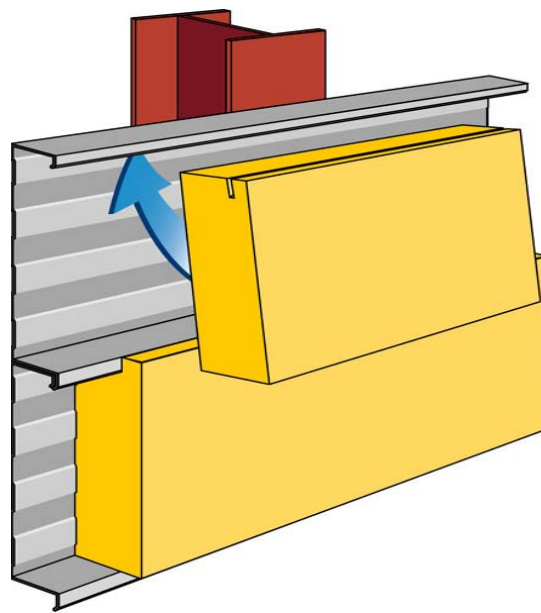
Figure 14 - Principe de mise en œuvre de l'isolant à l'intérieur du plateau
