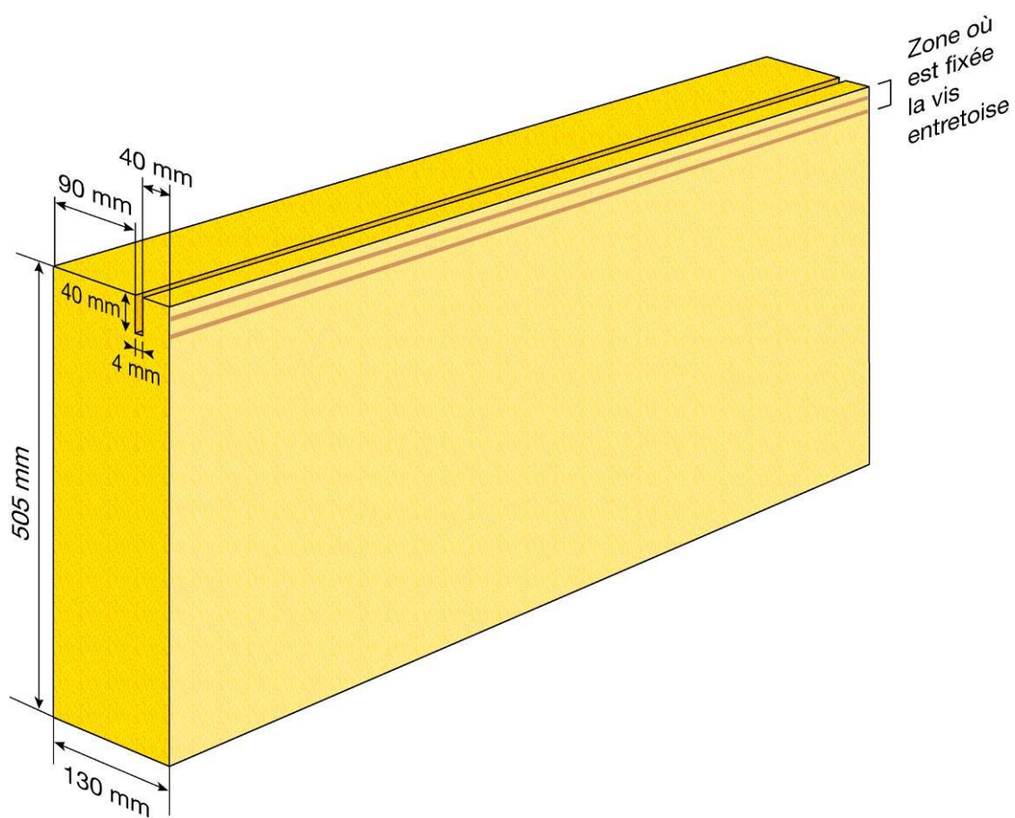
Figure 7 - Exemple de géométrie du Cladirol 35 ou Cladipan 32
