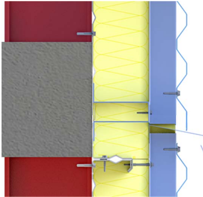
Figure 16 – Détail du fractionnement au droit des planchers pour la pose en zones sismiques
