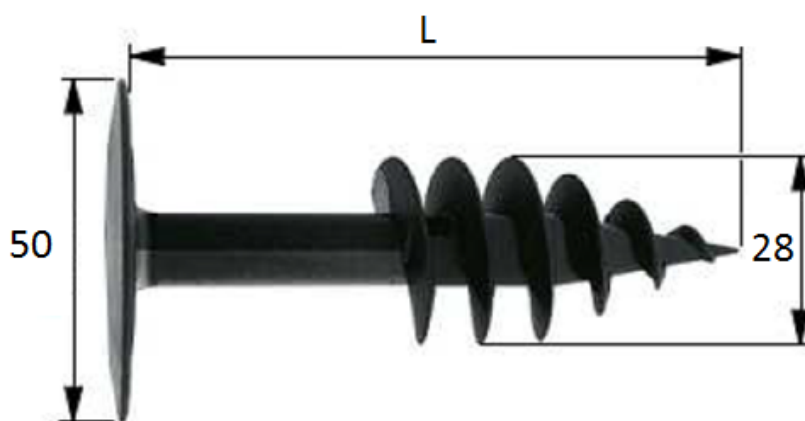
Figure 4 - Fixation SK-RB (Etanco) pour la fixation de l'Isobardage 32 en seconde couche
