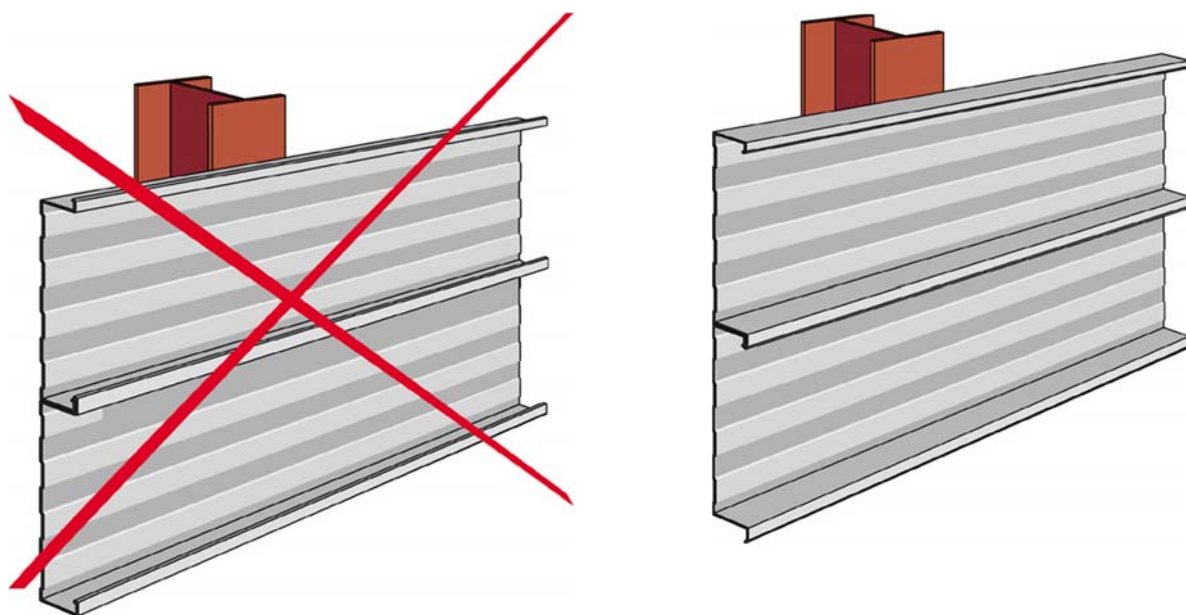
Figure 12 - Mise en œuvre des plateaux intérieurs
