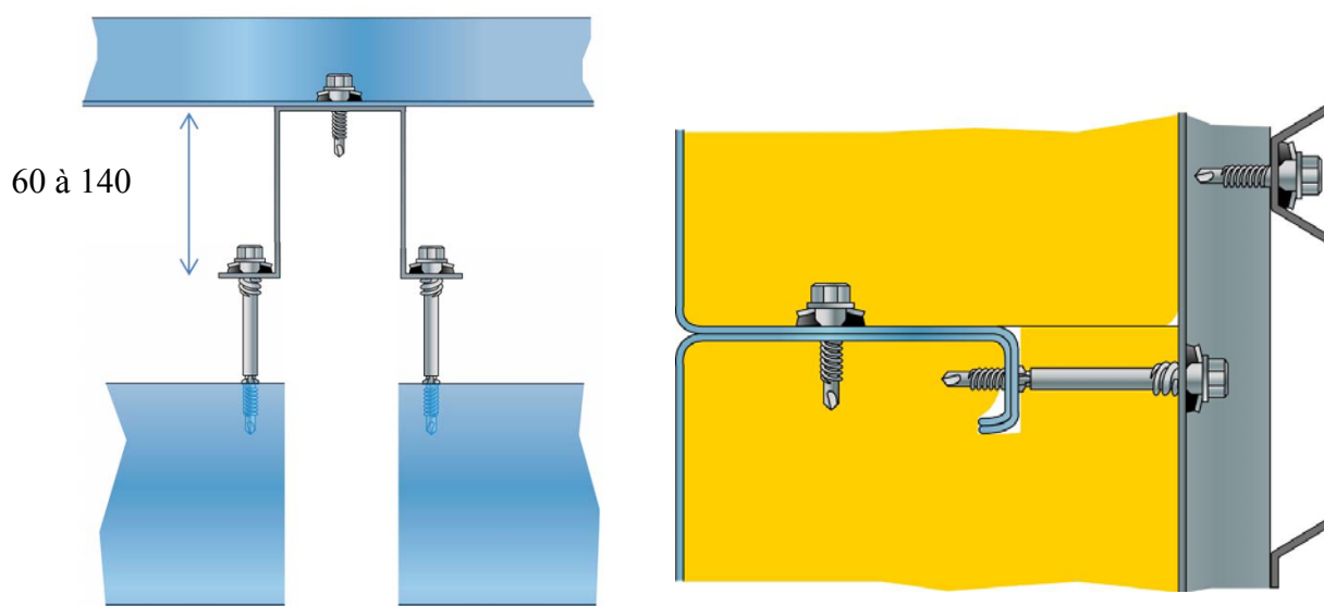
Figure 17 - Mise en œuvre d'une isolation en 2 couches
