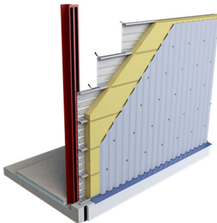
Figure 26 – Exemple de traitement des jonctions par joints compri-bandes
