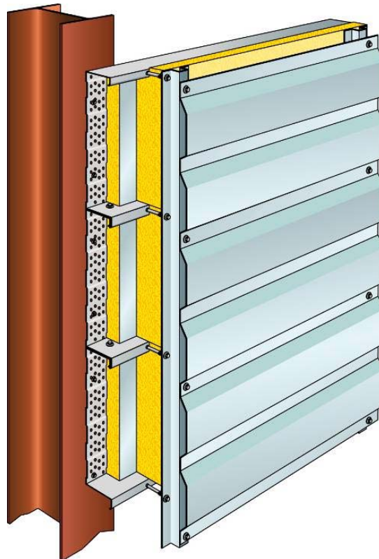
Figure 9 - Mise en œuvre du Cladacoustic (Bardage Horizontal)
