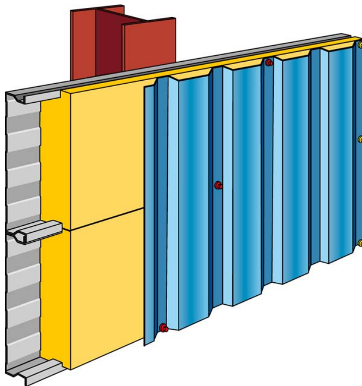
Figure 6 - Plateaux à lèvres caisson
