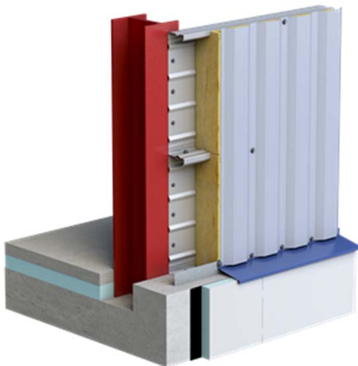
Figure 19 - Détail du pied de Bardage Vertical
