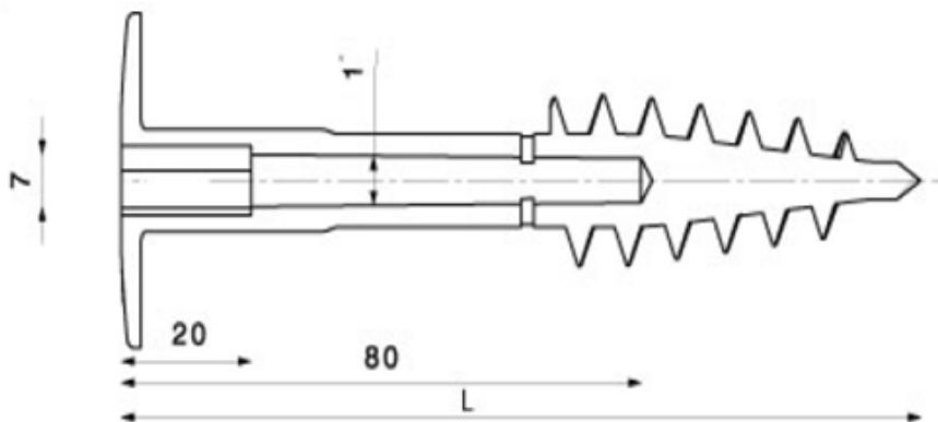
Figure 3 - Fixation RS-45/23 (SFS Intec) pour la fixation de l'Isobardage 32 en seconde couche
