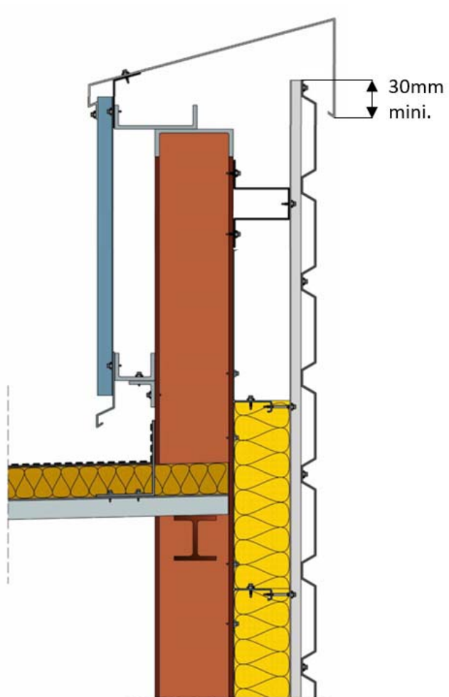
Exemple de solution avec ossature intermédiaire et sans profil de reprise de charge
