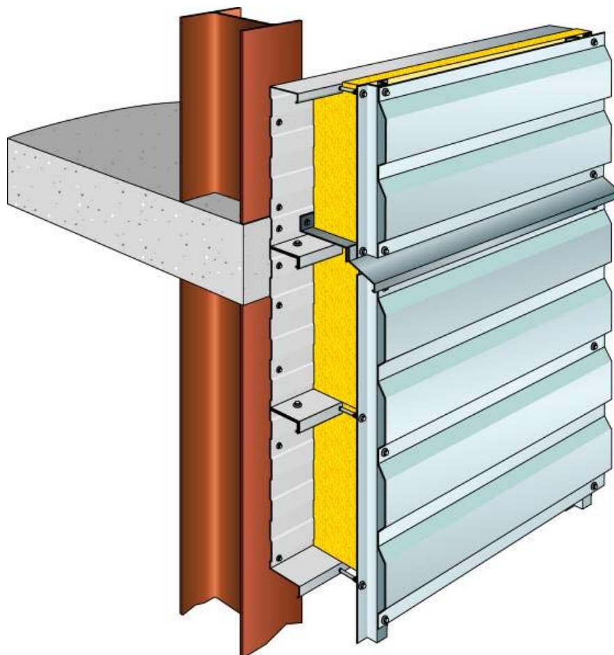
Figure 16bis – Fractionnement d'ossature au droit de chaque plancher en zone sismique avec profil de reprise de charge sur bardage horizontal
