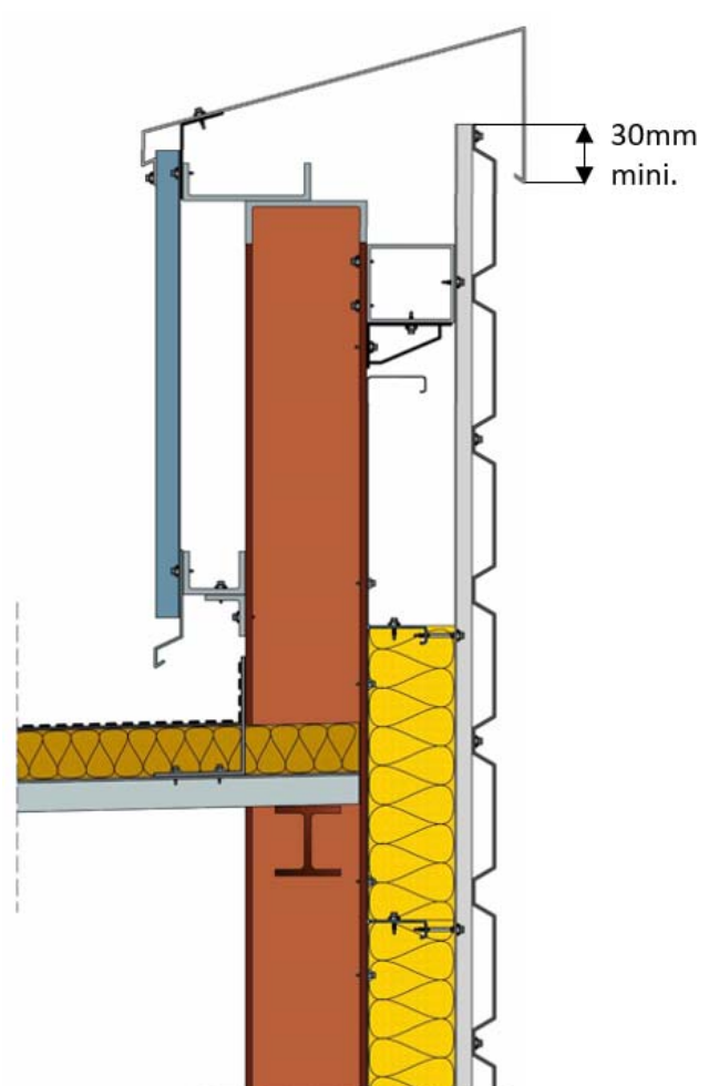
Exemple de solution avec ossature intermédiaire et avec un profil de reprise de charge
