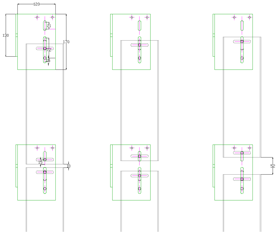
Figure PL6 Montage platine pour reprise de flèche et profilé
