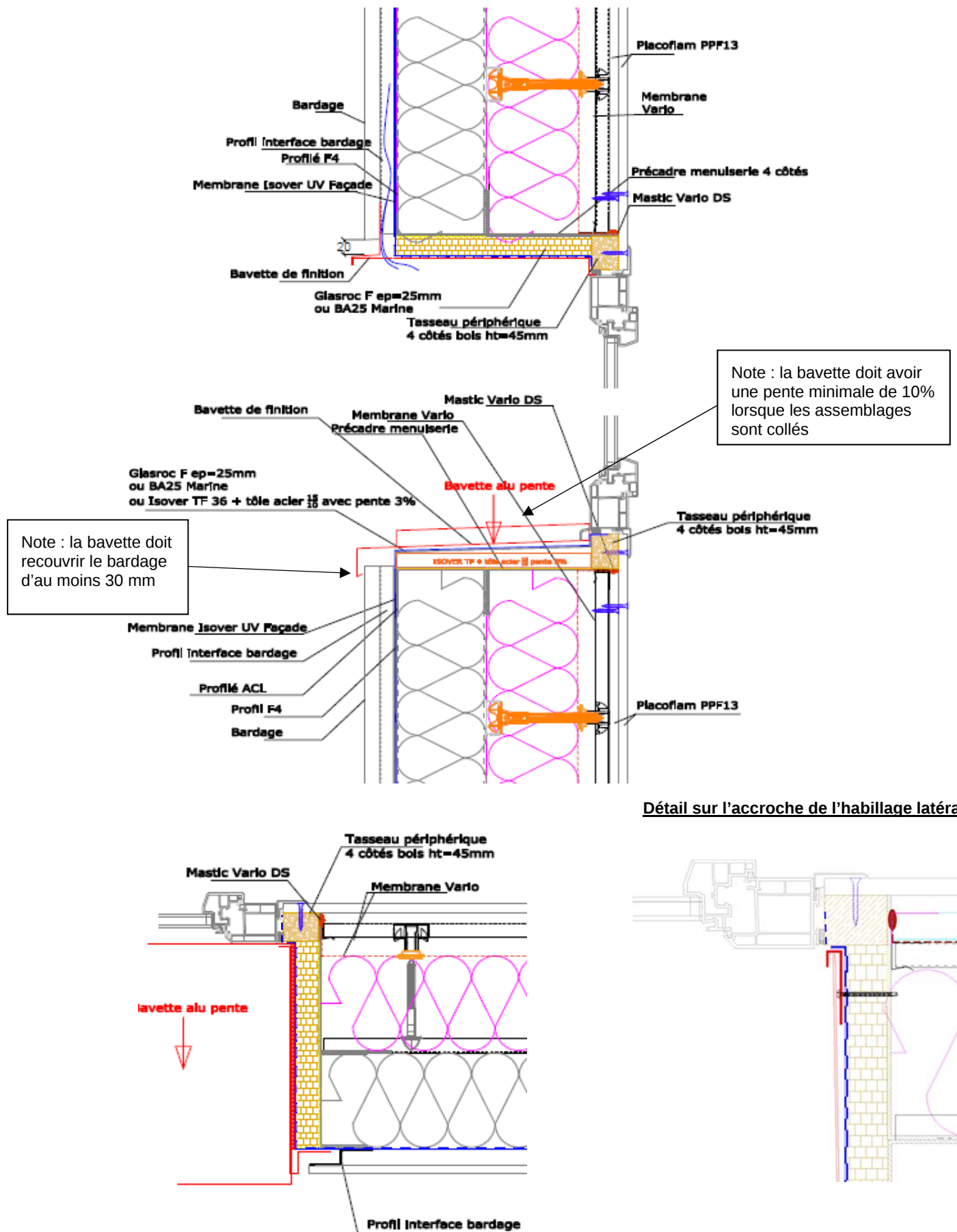
Figure AX 8 Coupe sur menuiserie avec habillage et détail sur l'accroche de l'habillage latéral
