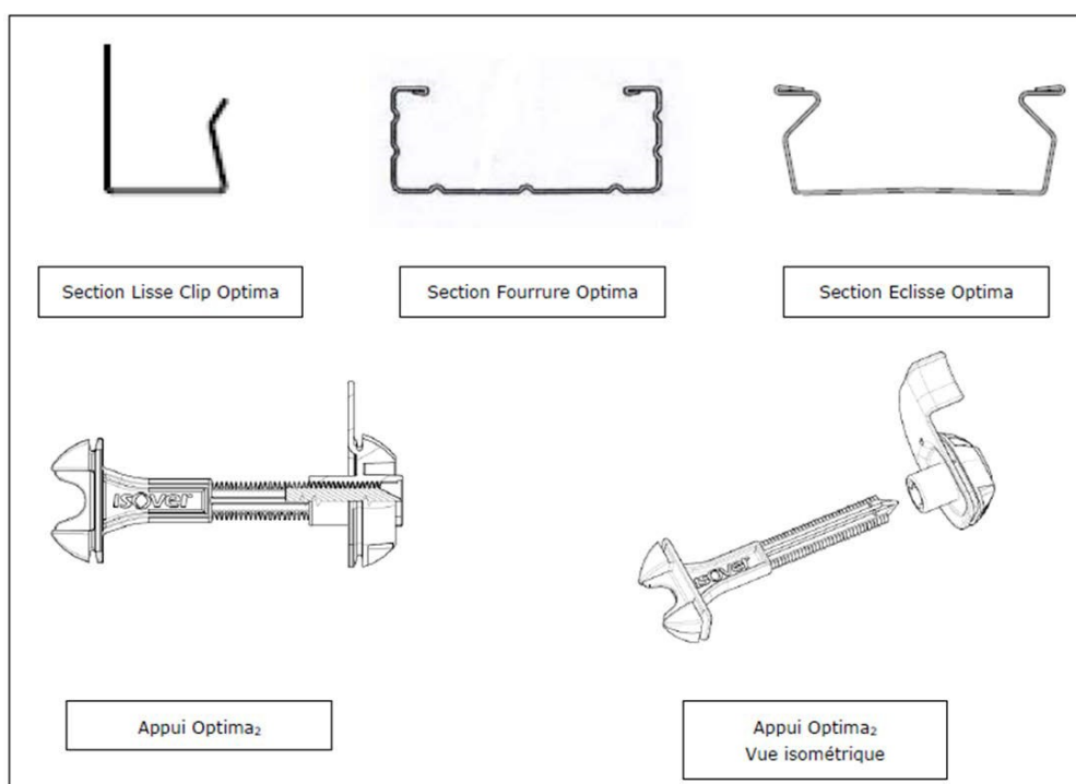
Figure AX 5 Eléments du système OPTIMA
