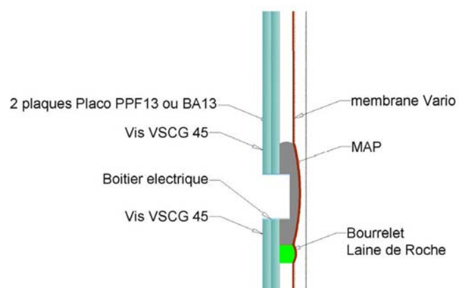
Figure AX 6 Boitier d'encastrement feu et son montage
