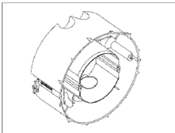
Figure AX 6 Boitier d'encastrement feu et son montage
