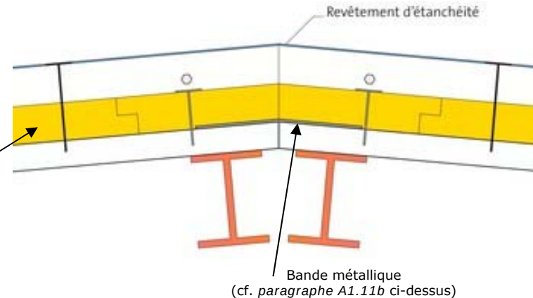
Figure 6 – Principe de jointoiement du procédé Stisolétanch® Protect avec élément porteur tôle d'acier nervurée, sur appui double du faîtage ou arêtier
