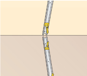
1 POSE DES FOURRURES, LISSES ET APPUIS
