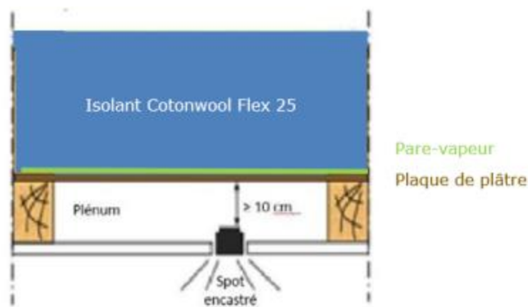
Figure 3 – Spot encastré dans un plénum
